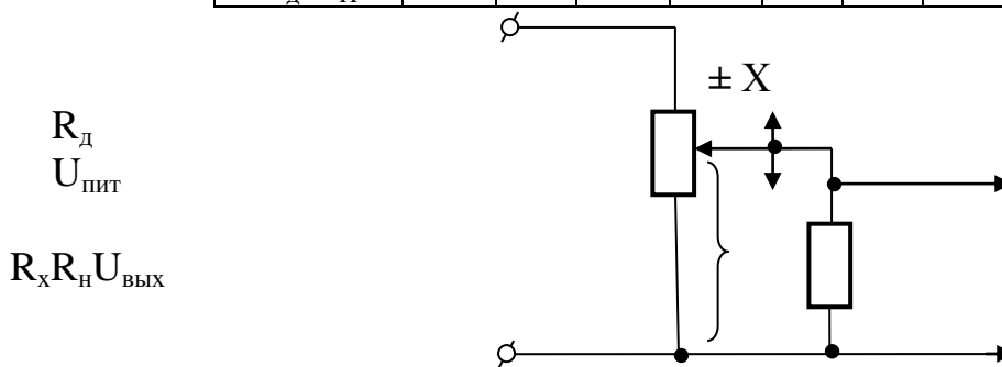
Рис. 1. Схема включения резистивного датчика
